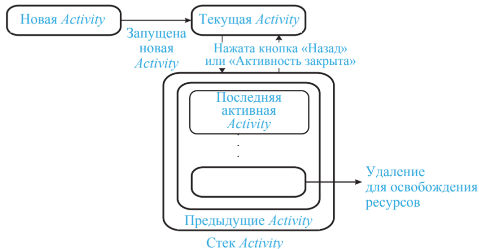
Рис. 3.1. Стек активностей
